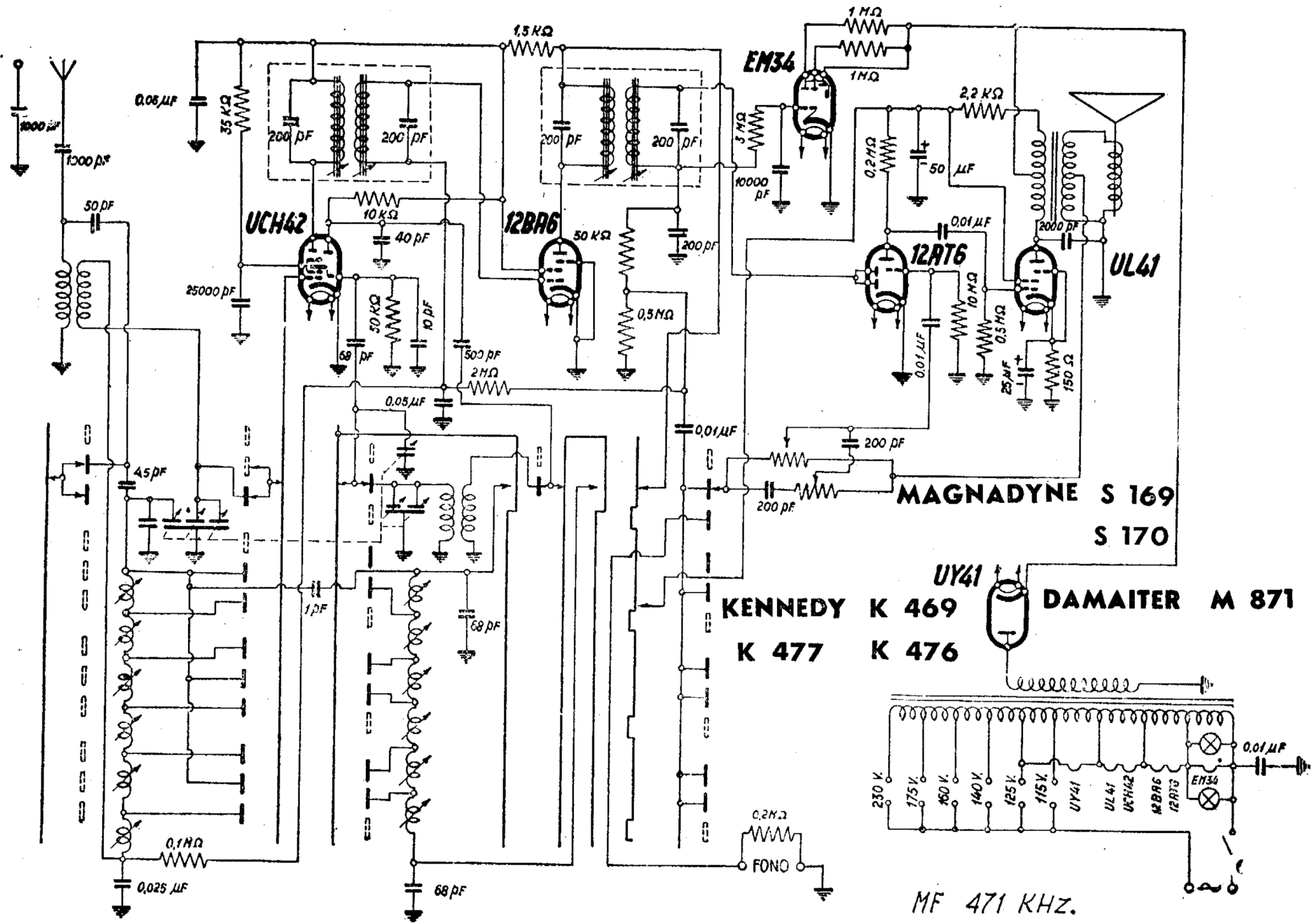
MAGNADYNE RADIO - Modd. MAGNADYNE S 169, S 170, DAMAITER M 871, KENNEDY K 469, K 476 e K 477. Una gamma ad onde medie e sei bande allargate ad onde corte e cortissime. Media frequenza 471 kc/s.
